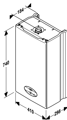
SEMIA F 21 – wymiary w mm
