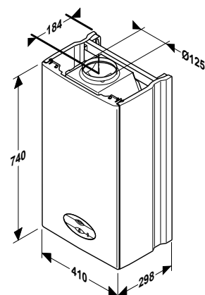
SEMIA C 24 – wymiary w mm
